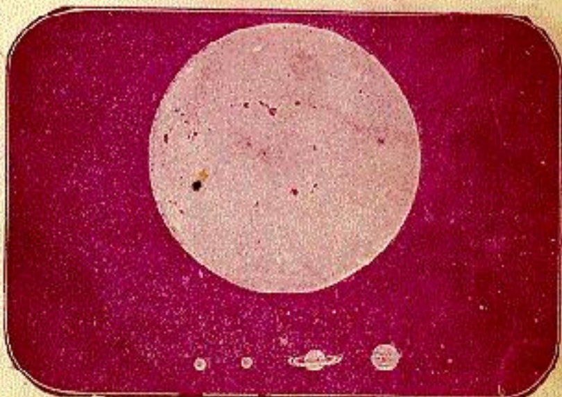
TAMANO DEL SOL COMPARADO CON LOS PLANETAS
