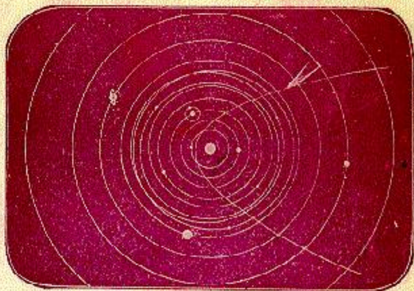
NUESTRO SISTEMA PLANETARIO
